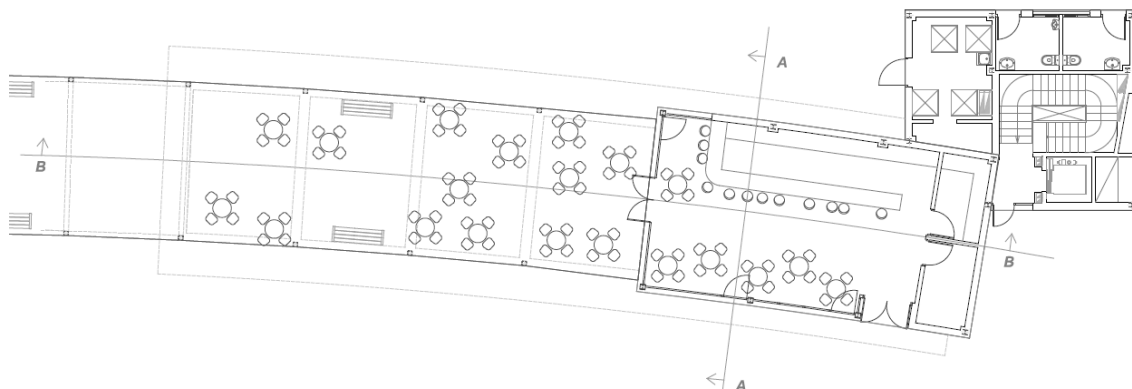
Plànol de planta de la plaça per als vianants on se situa la cafeteria.
