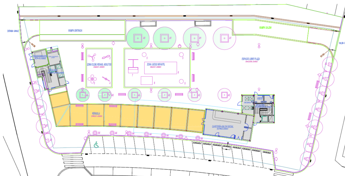
Plànol de planta de la plaça per als vianants on se situa la cafeteria.
