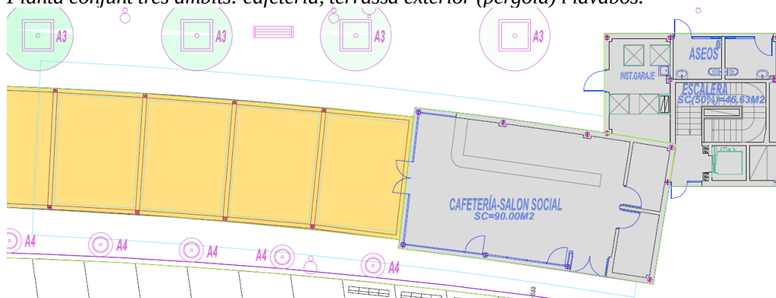
Planta conjunt tres àmbits: cafeteria, terrassa exterior (pèrgola) i lavabos.
